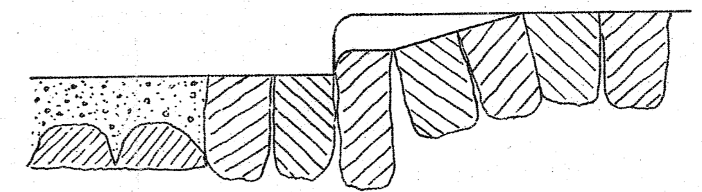
Overkørsel. 1:10.
