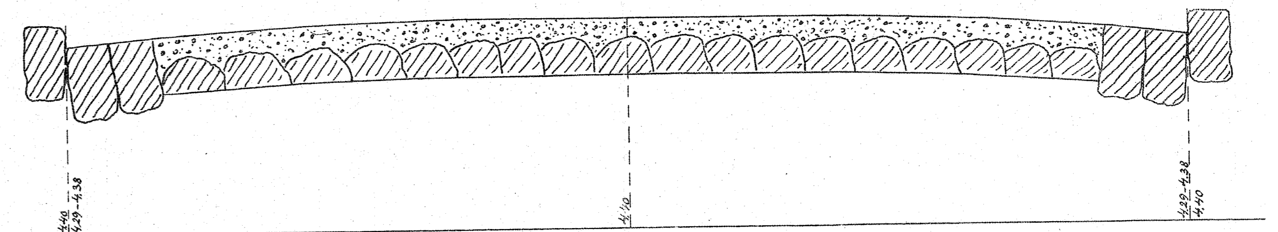
Tværsnit af Køresti. 1:10
